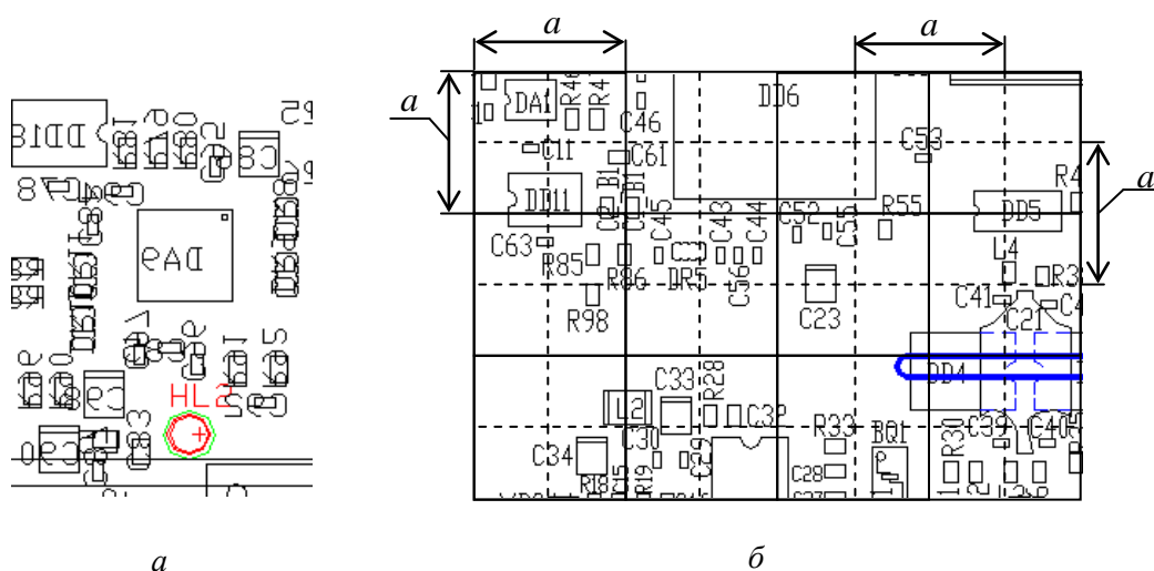
Рисунок 1: Разбиение печатной платы на зоны:
