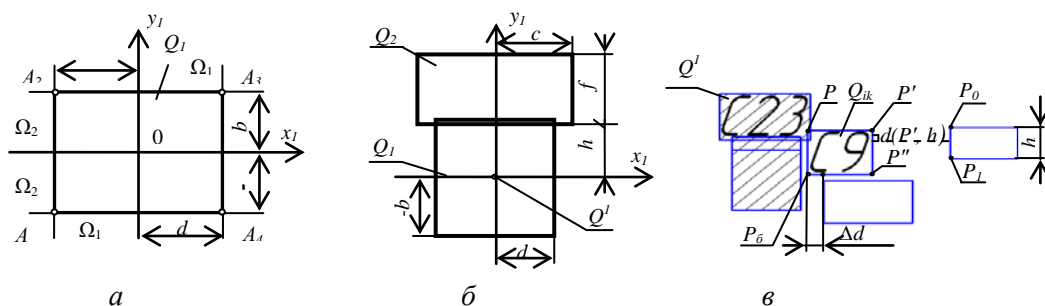
Рисунок 3: Определение уравнения прямоугольника области Q^l , и траектории движения текстов обозначений элементов печатной платы
